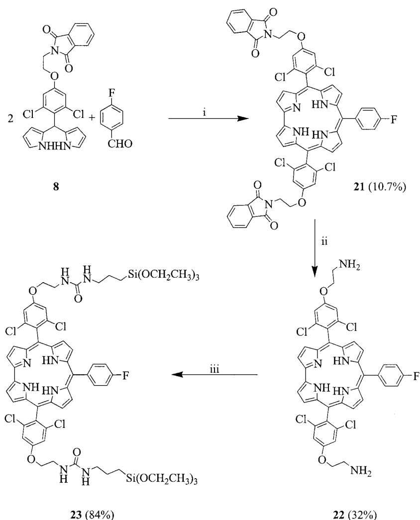
Scheme 6. i) 1: TFA, CH 2 Cl 2 ; 2: DDQ. ii) NH 2 NH 2 , H 2 O, EtOH. iii) IPTES (2.5 equiv.), i Pr 2 NEt (6 equiv.), MeCN, 12 h.
