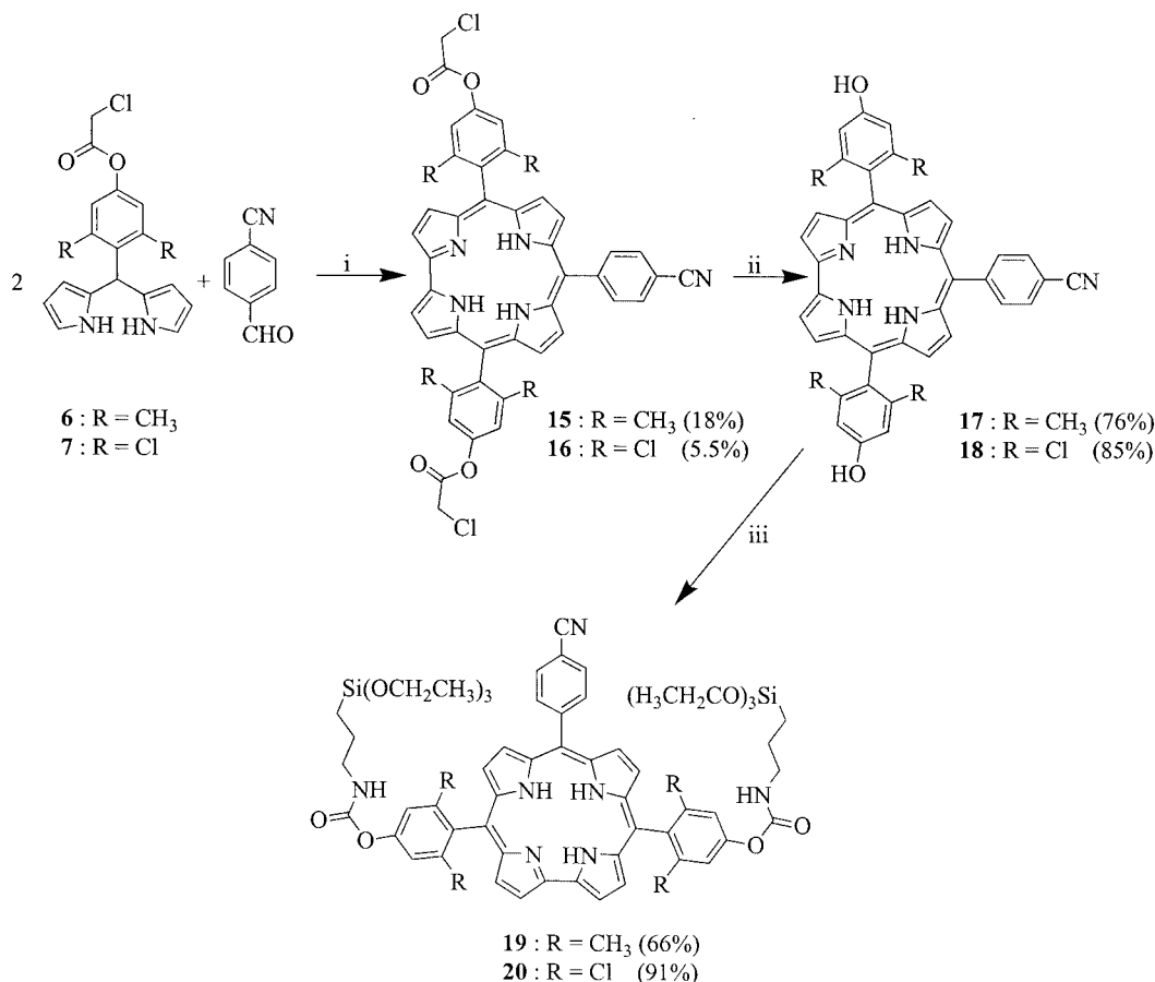
Scheme 5. i) 1: TFA, \text{CH}_2\text{Cl}_2 ; 2: DDQ. ii) \text{PhCH}_2\text{NH}_2 , THF, EtOH. iii) IPTES (8 equiv.), i\text{Pr}_2\text{NEt} (8 equiv.), MeCN, 7 days.
