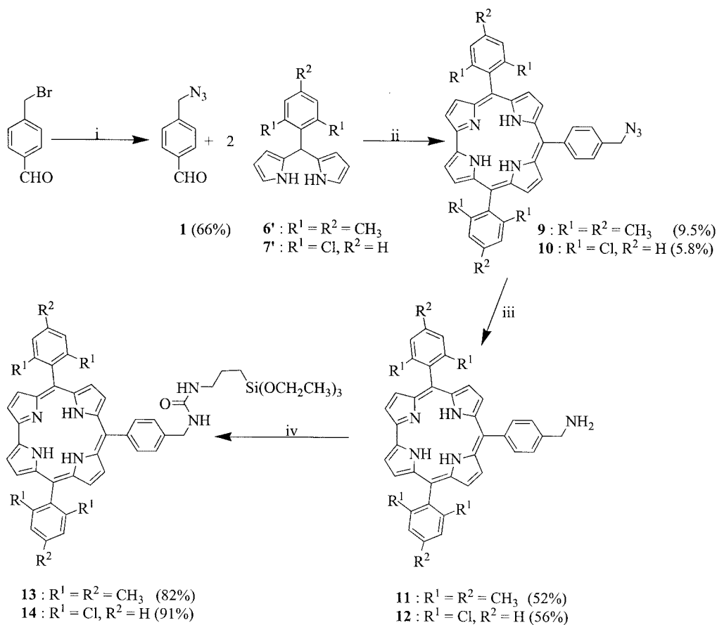
Scheme 2. i) \text{NaN}_3 , acetone, \text{H}_2\text{O} . ii) 1: TFA, \text{CH}_2\text{Cl}_2 ; 2: DDQ. iii) \text{PPh}_3 , \text{H}_2\text{O} , THF. iv) IPTES (1.05 equiv.), MeCN, 12 h.
