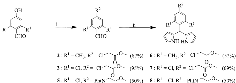
Scheme 4. i) (2) 1: \text{NEt}_3 , THF; 2: \text{ClCOCH}_2\text{Cl} . (3) 1: i\text{Pr}_2\text{NEt} , THF; 2: \text{ClCOCH}_2\text{Cl} . (5) N -(2-bromoethyl)phthalimide, \text{K}_2\text{CO}_3 , MeCN. ii) pyrrole, TFA.
